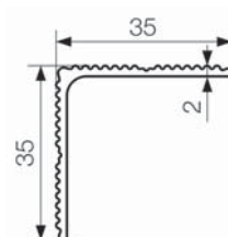
Wymiary aluminiowej listwy wykończeniowej (mm)
