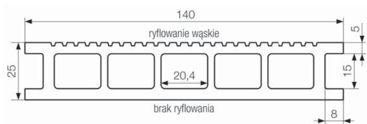
Wymiary deski (mm)
