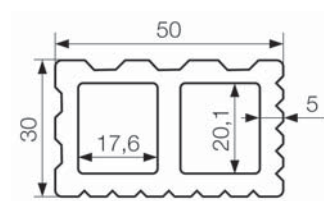
Wymiary legara (mm)
